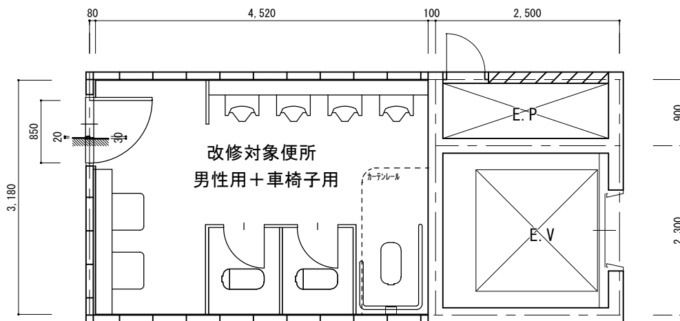
現況図 (西側トイレ)
